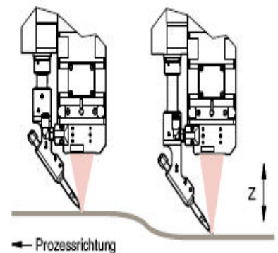
Fokusschnachführung in Z-Richtung
